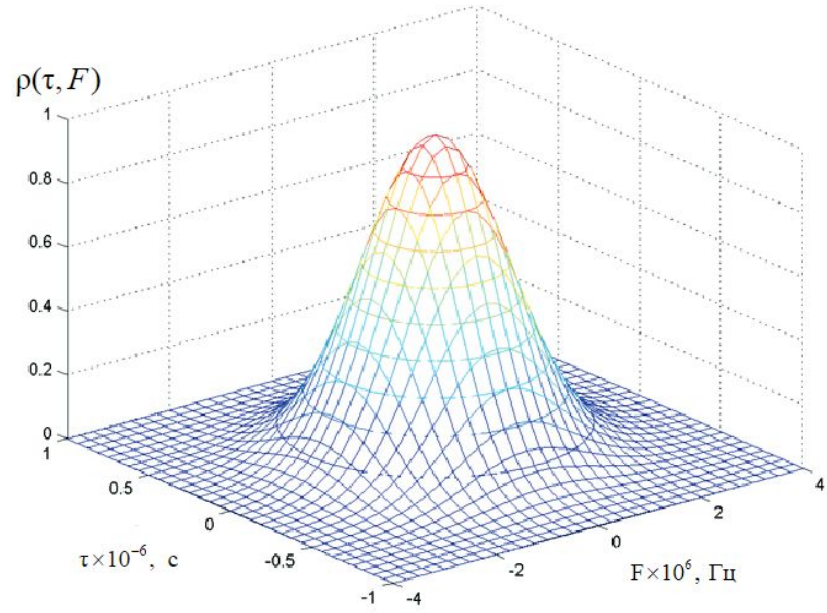
Изображение двумерной автокорреляционной функции одиночного радиоимпульса
