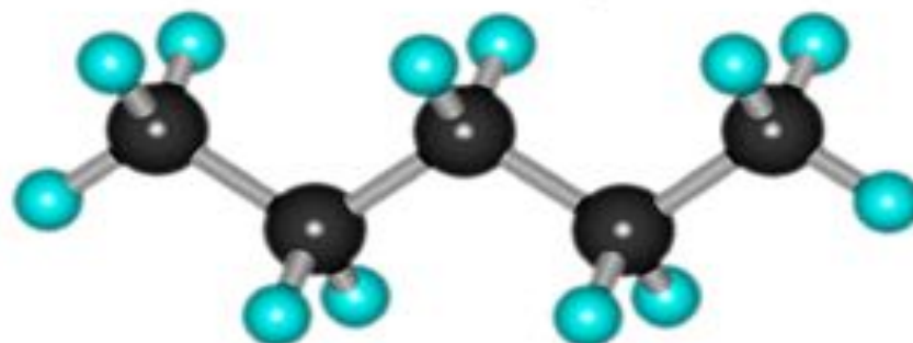
Модель молекулы
