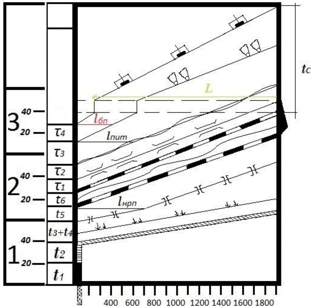
выправка пути машиной ВПО-3000
