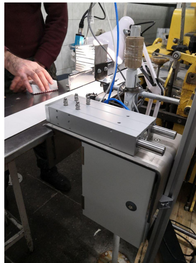
Автоматический выбраковщик на линии фасовки масла
