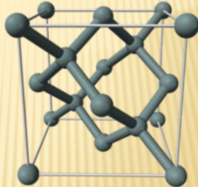
Кристаллическая структура кремния.
