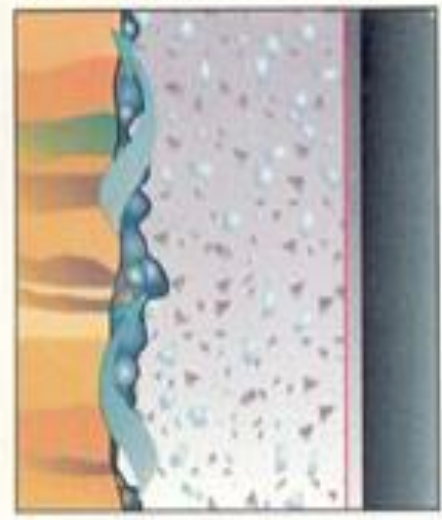
Некачественное удаление бур. р-ра / фильтрац. корки
