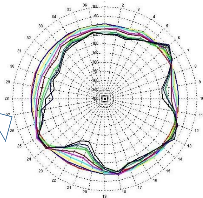
График отклонений образующих стенки резервуара от вертикали (горизонтальное сечение)
