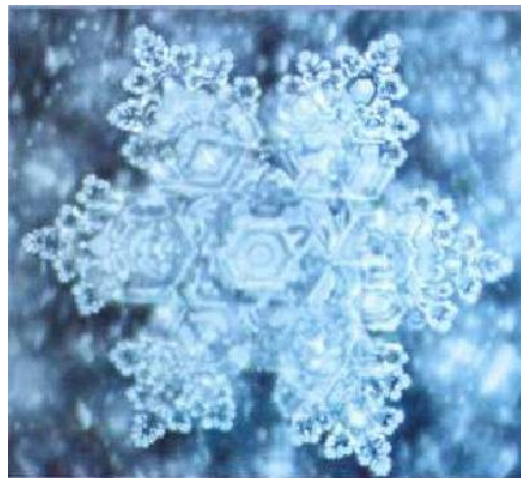
Кристаллы льда
