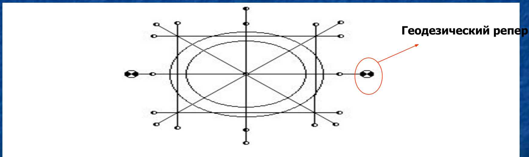
Рис. 2. Схема размещения знаков закрепления главных и основных осей при строительстве зданий круглой конфигурации
