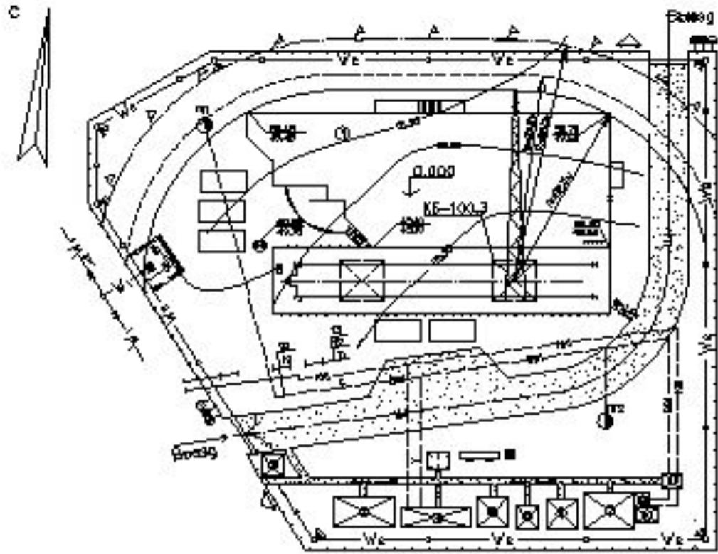
СТРОИТЕЛЬНЫЙ ГЕНЕРАЛЬНЫЙ ПЛАН ОБЪЕКТА И 1:200
