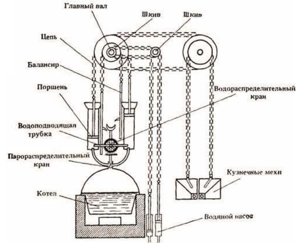
Схема паровой машины И.И. Ползунова
