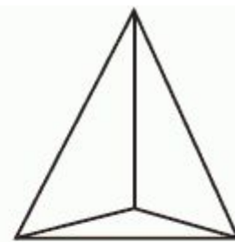
Тетраэдр
