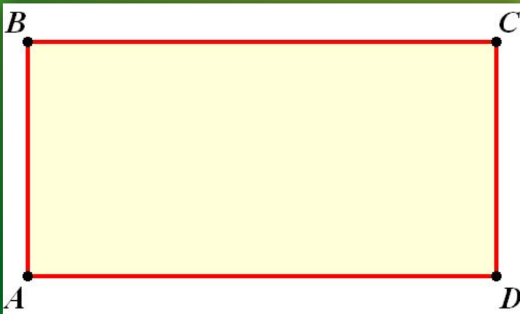
Прямоугольник ABCD
