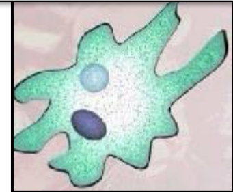
Амеба (одноклеточное)
