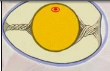
Яйцеклетка
