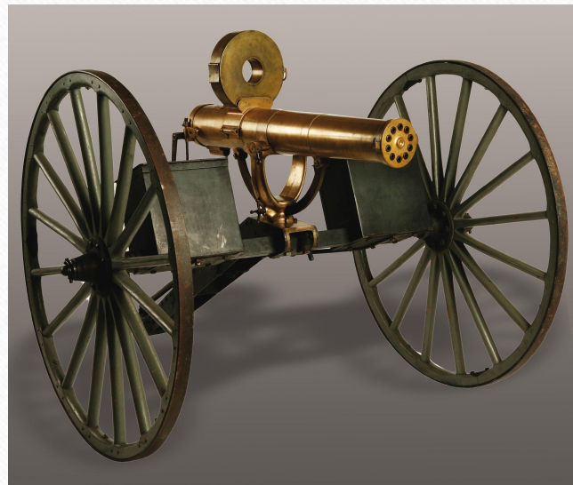
Картечьница (пулемет) Гатлинга
