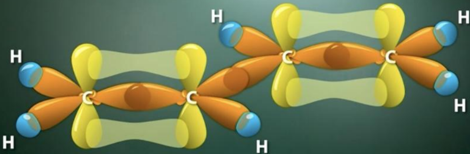
Молекула бутадиена
