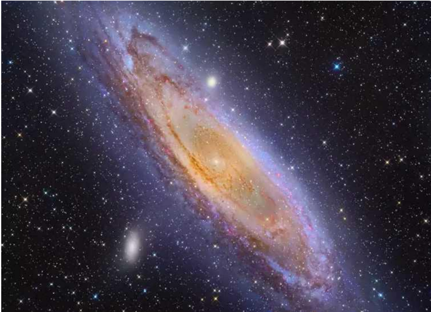
Туманность Андромеды
