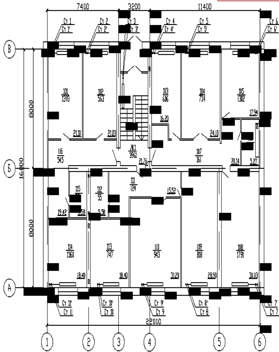
Рисунок Б2 – Пример оформления плана этажа при двухтрубном присоединении отопительных приборов
