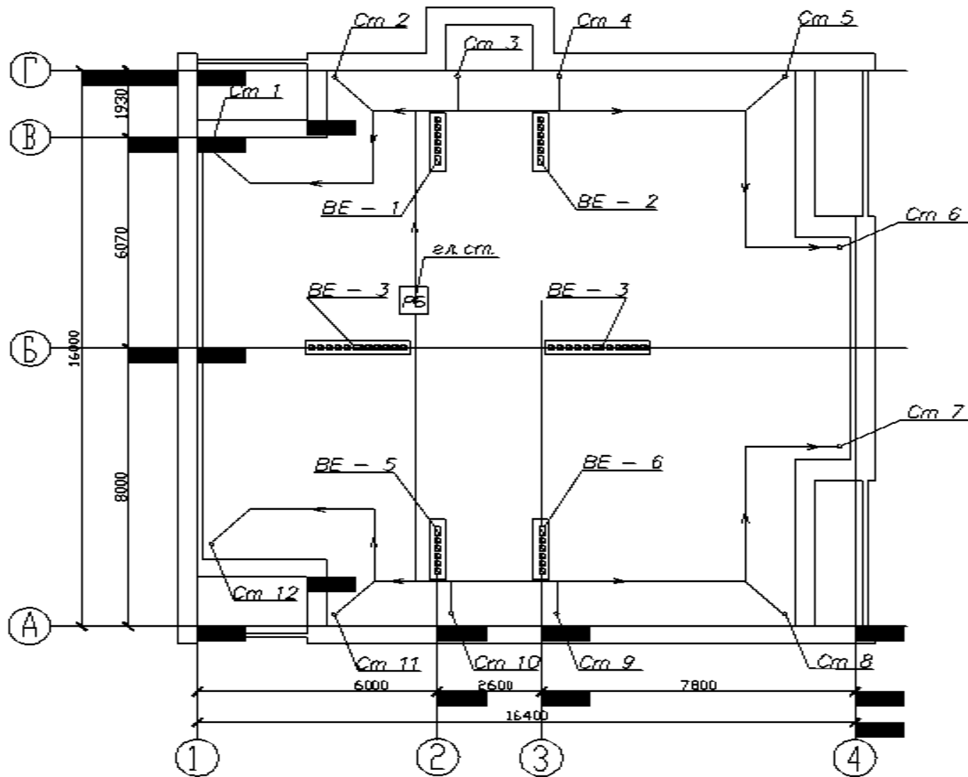
Рисунок Бб – Пример оформления плана чердака при тупиковой схеме движения теплоносителя и верхней разводке
