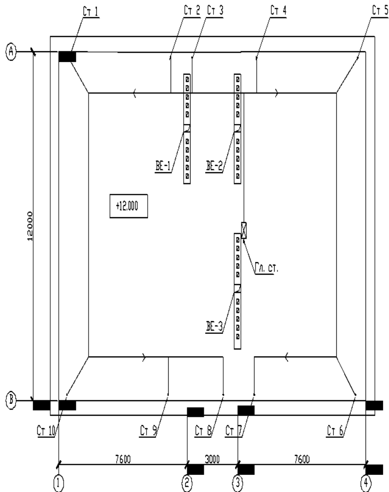
Рисунок Б8 – Пример оформления плана чердака при попутной схеме движения теплоносителя и верхней разводке
