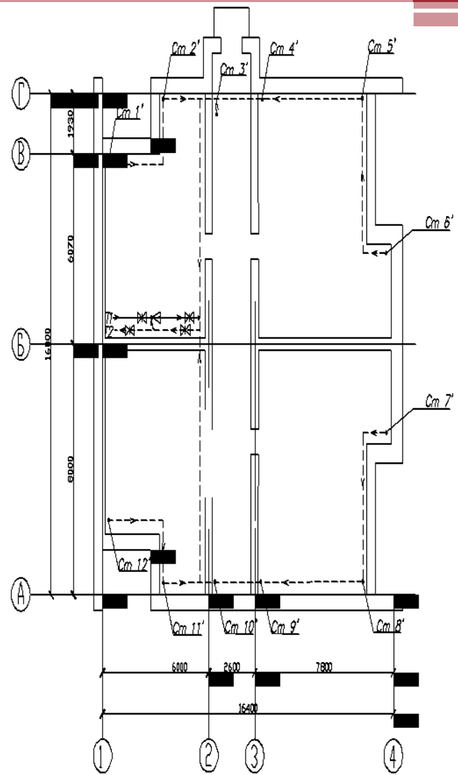
Рисунок Б5 – Пример оформления плана подвала при тупиковой схеме движения теплоносителя и верхней разводке
