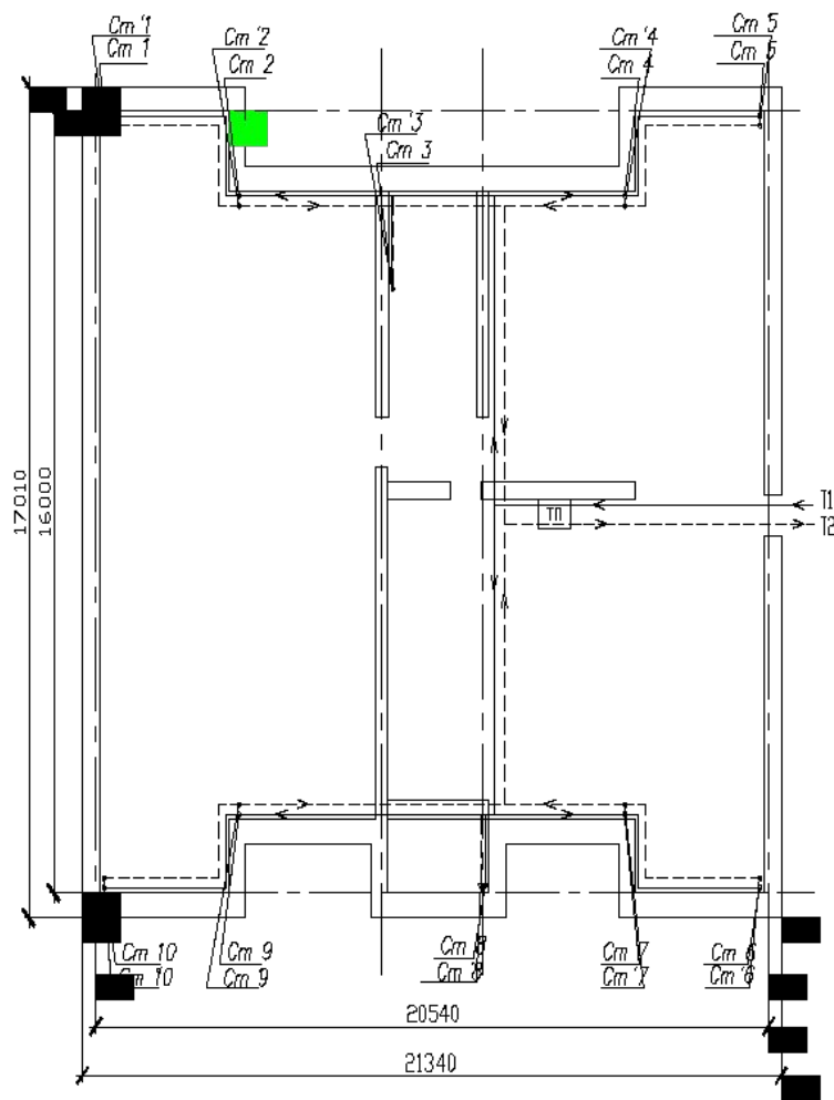
Рисунок Б3 – Пример оформления плана подвала при тупиковой схеме движения теплоносителя и нижней разводке
