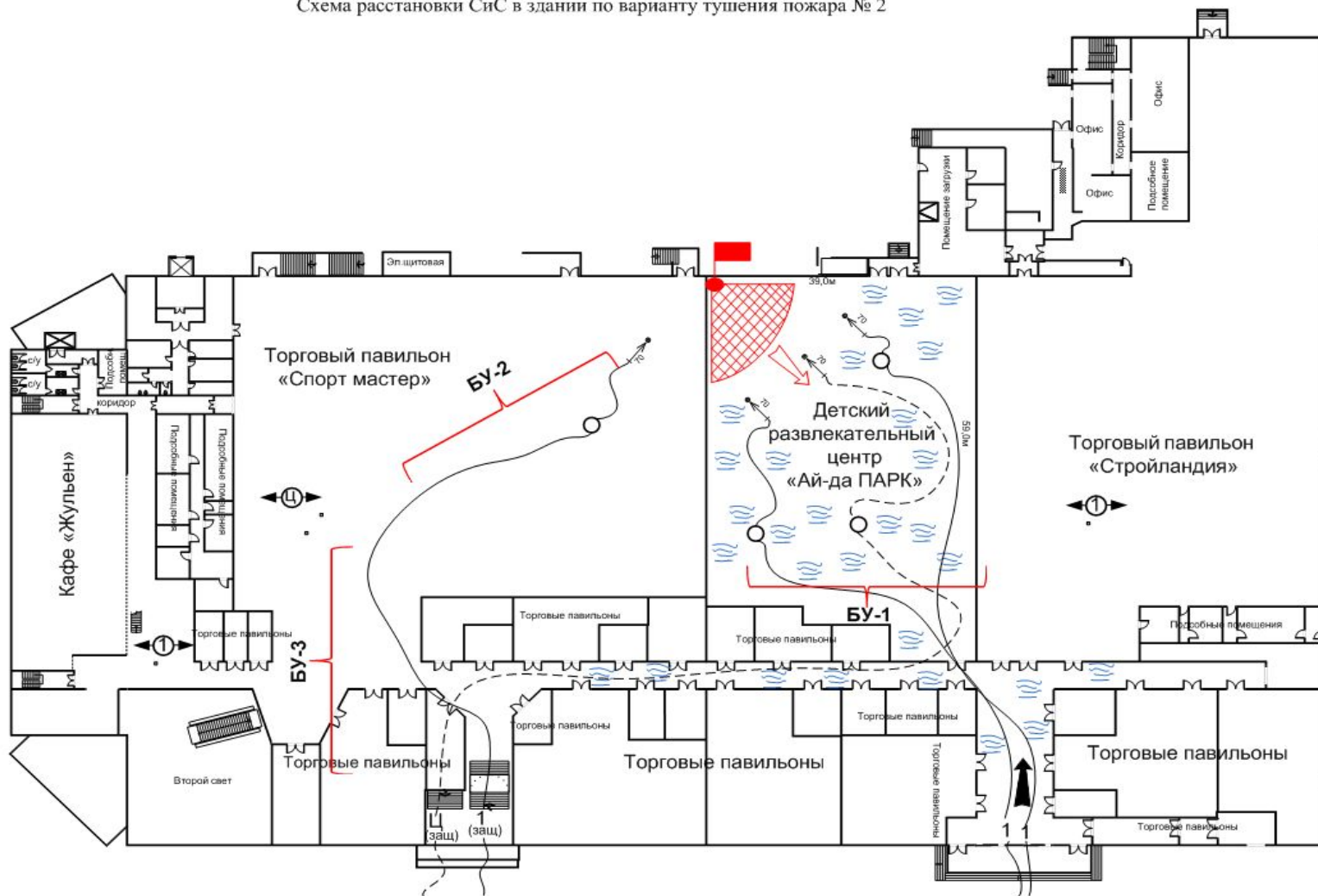
Схема расстановки СИС в здании по варианту тушения пожара № 2
