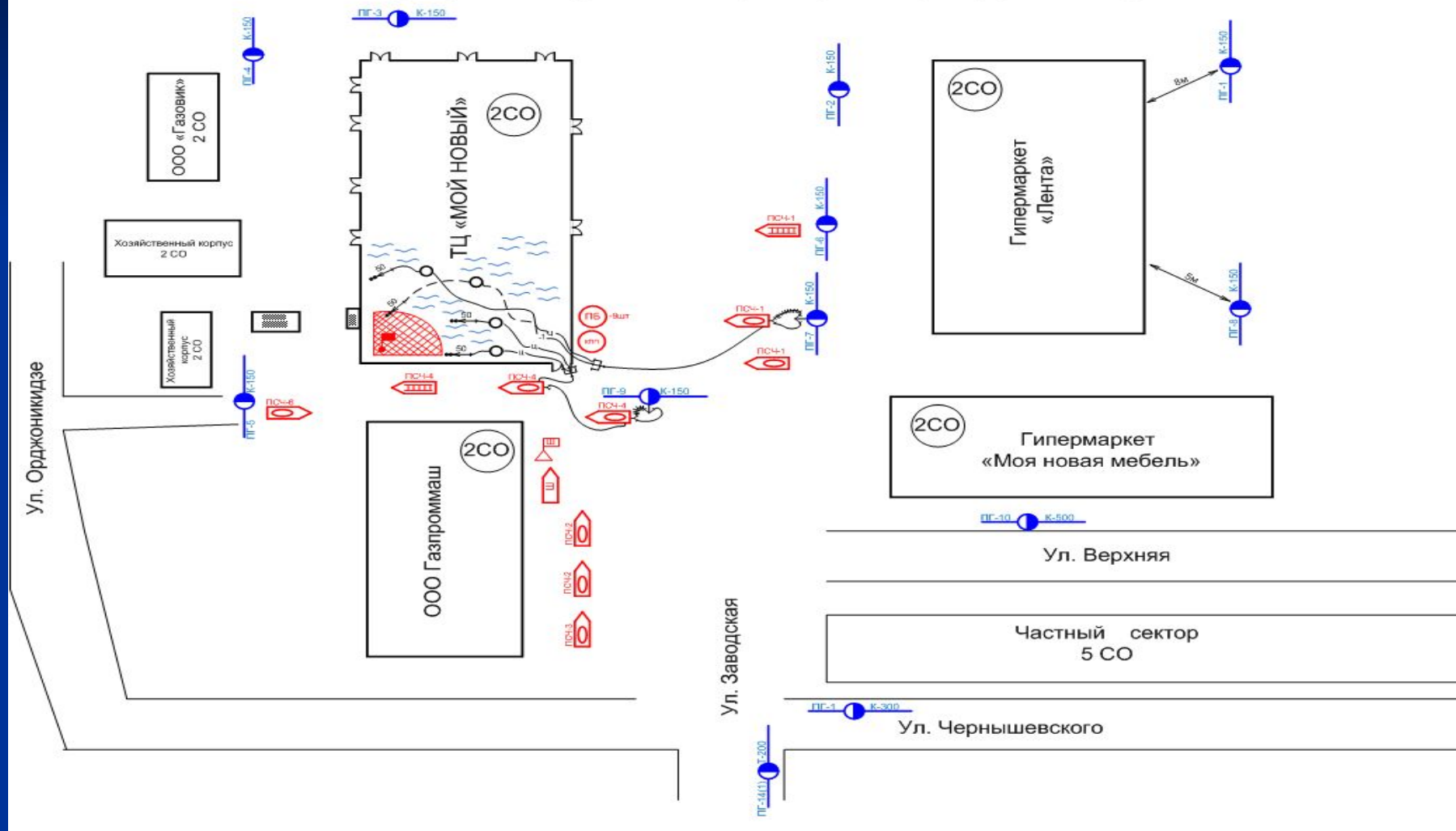
Схема развёртывания подразделений пожарной охраны по варианту тушения пожара № 1
