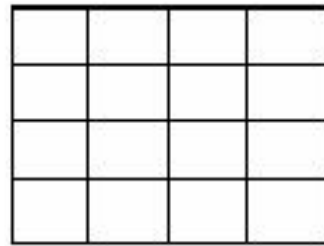
ДВУМЕРНЫЙ МАССИВ
