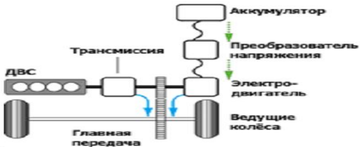
Рисунок 2 — Параллельная схема.
