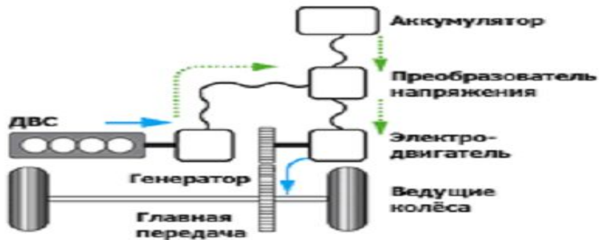
Рисунок 1 — Последовательная схема.
