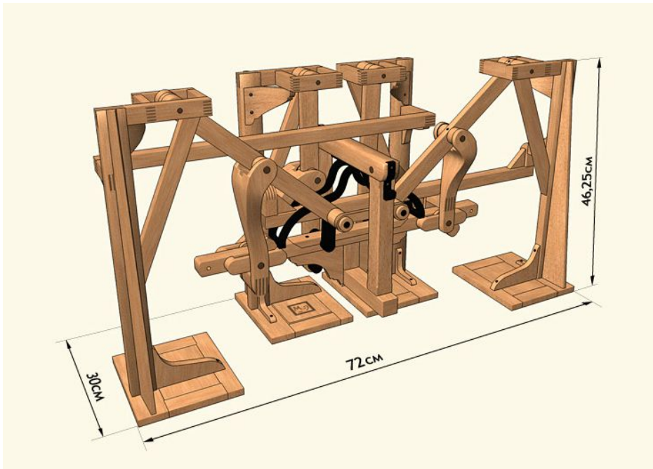
2) Стопоходящая машина
