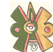
Землетрясение
