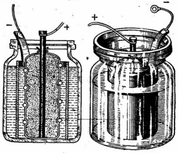
Схема гальванической установки
