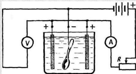
Схема гальванической установки
