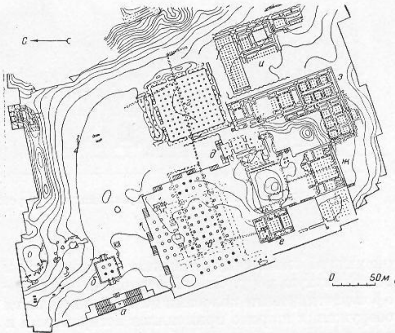
53. Город Персеполь, VI—IV вв. до н. э. Генеральный план. Террасы дворцов: а — лестница; б — пропилеи Ксеркса; в — ападана Дария и Ксеркса; г — «Зал ста колонн»; д — трипилон; е — дворец Дария; ж — дворец Ксеркса; з — «гарем» Ксеркса; и — сокровищница
