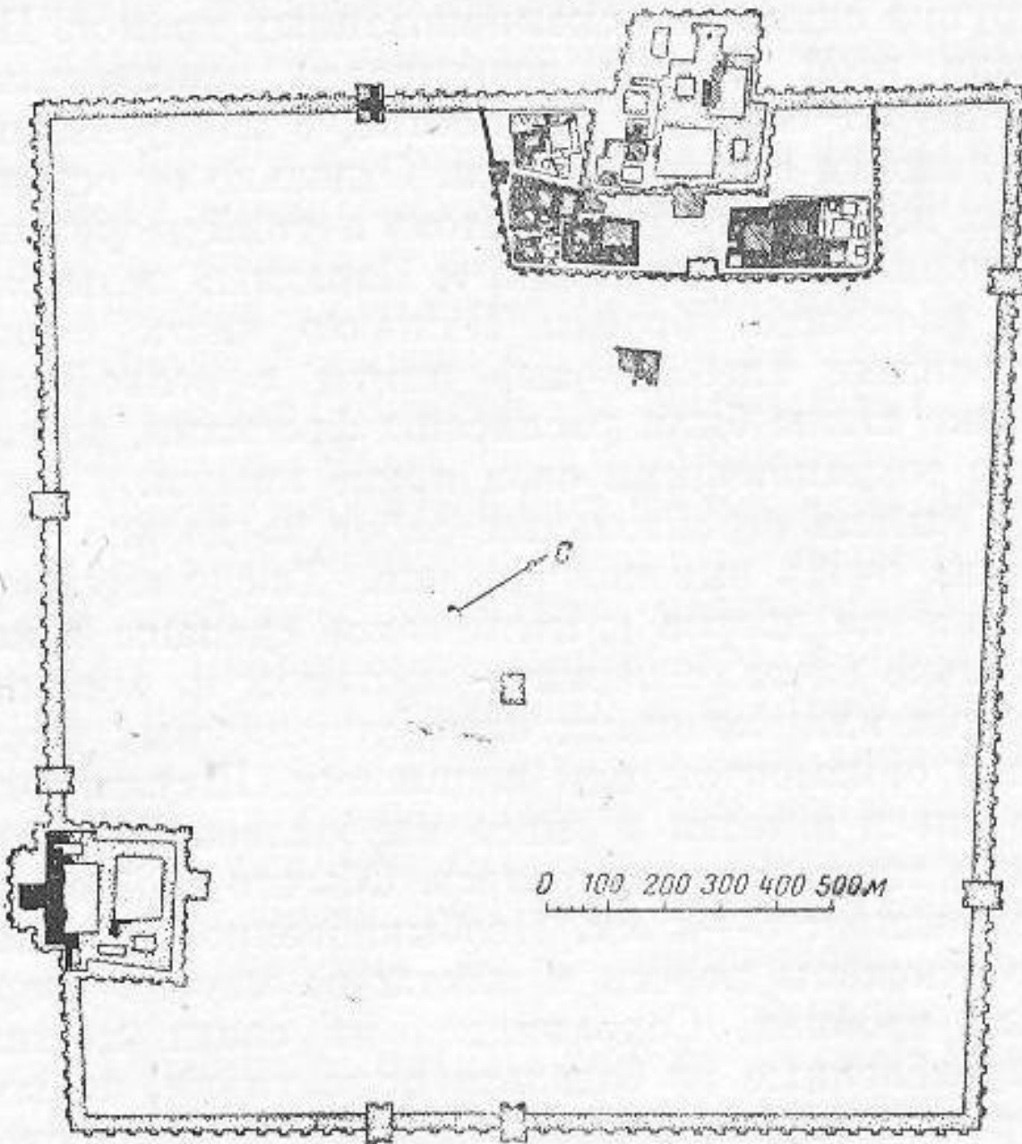
40. Город Дур-Шаррукин, 711—707 гг. до н. э. План
