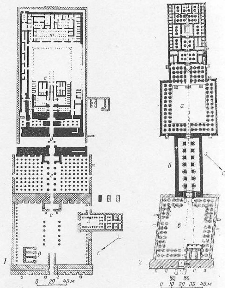
72. 1 — храм Амона в Карнаке, начало II тысячелетия — I в. до н. э. План: а — большой двор; б — храм Рамсеса III; в — храм Сети II; г — гипостильный зал; д — двор; е — развалины храма Среднего царства; ж — храм Тутмоса III. 2 — храм Амона в Луксоре, XV — середина XIII в. до н. э. План: а — храм Аменхотепса III; б — колоннада Аменхотепса III; в — двор Рамсеса II
