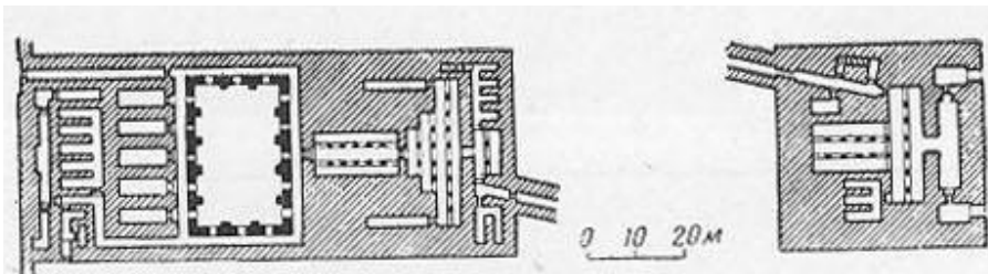
62. Заупокойный храм при пирамиде Хефрена в Гизе. Планы заупокойного храма и входного зала
