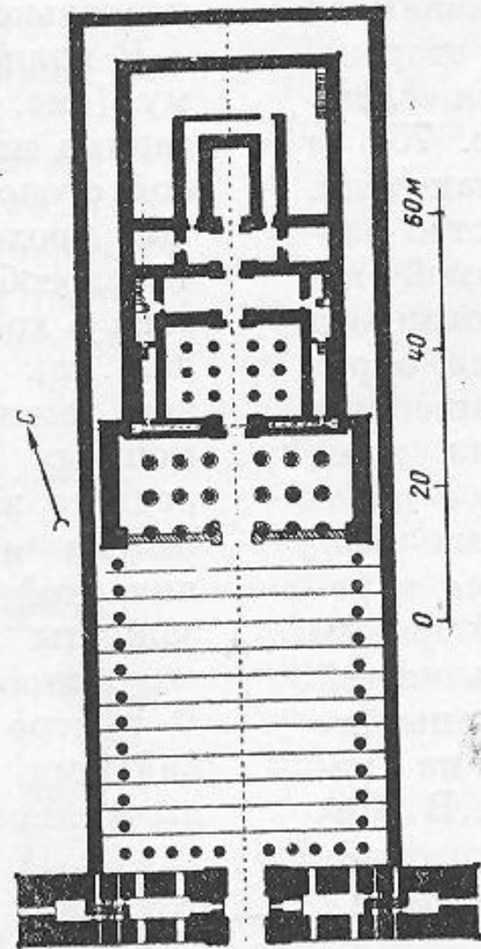
77. Храм Гора в Эдфу, 237 — 57 г. до н. э. План
