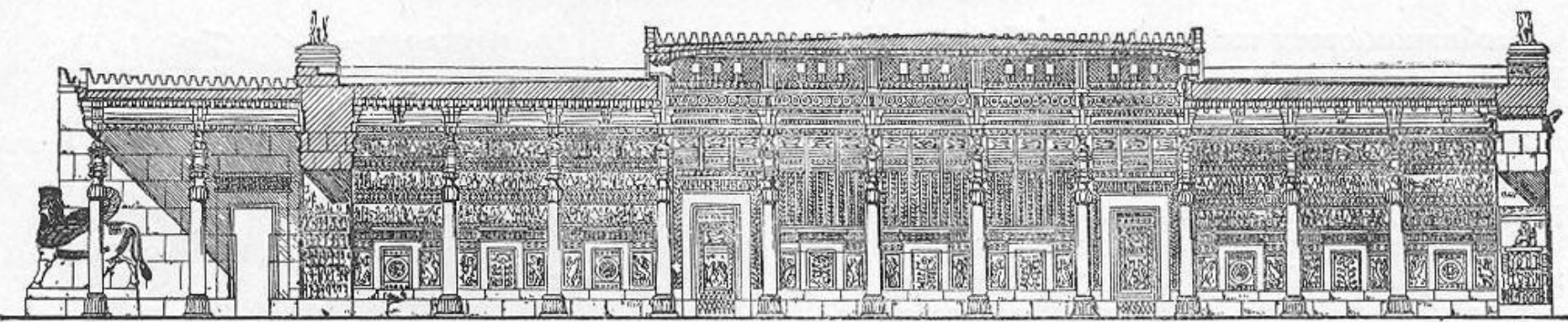
54. «Зал ста колонн» (сокровищница) в Персеполе, VI—V вв. до н. э. Разрез. Реконструкция Шипье
