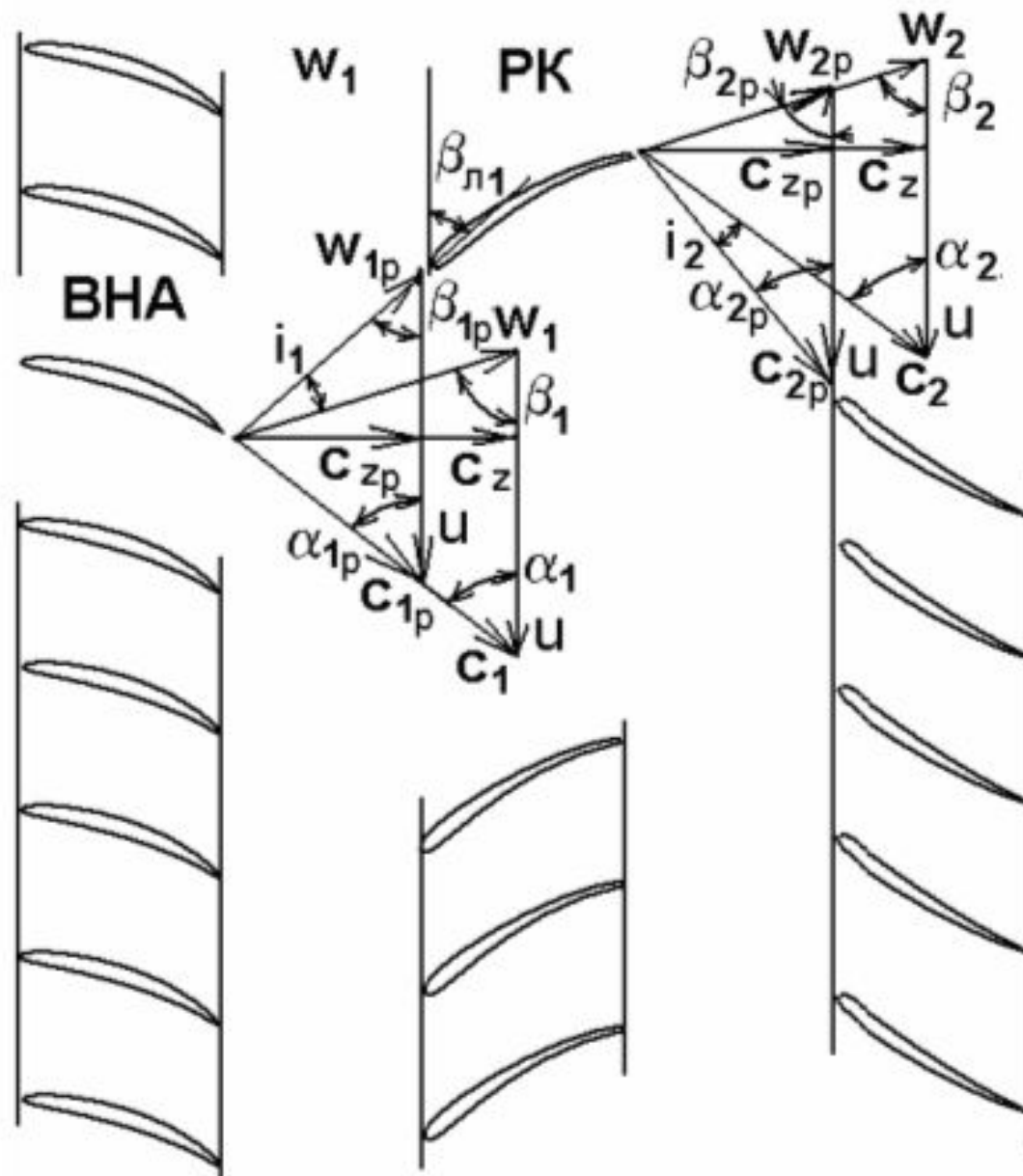
Треугольники скоростей на входе и выходе ПК осевого компрессора при изменении режима работы (индекс «р» - расчётный режим)
