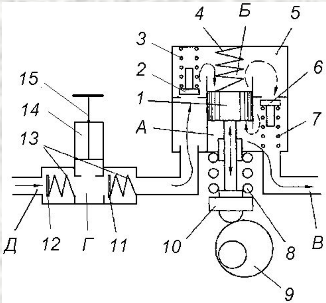
Схема работы топливopодкачивающего и топливopокачивающего насосов
