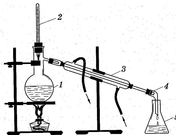
Рис. 2.2. Прибор для прямой перегонки жидкостей
