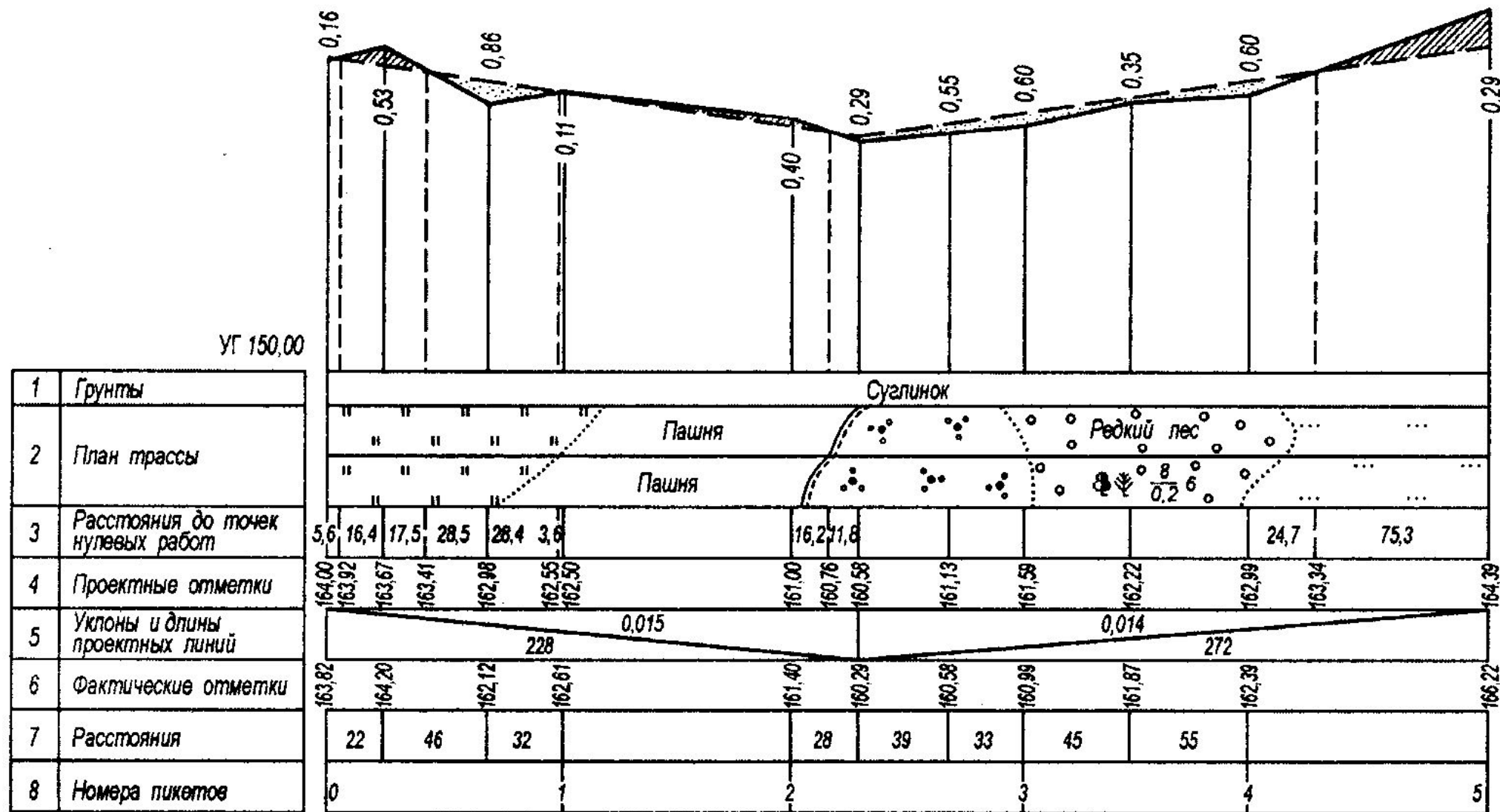
Продольный профиль
