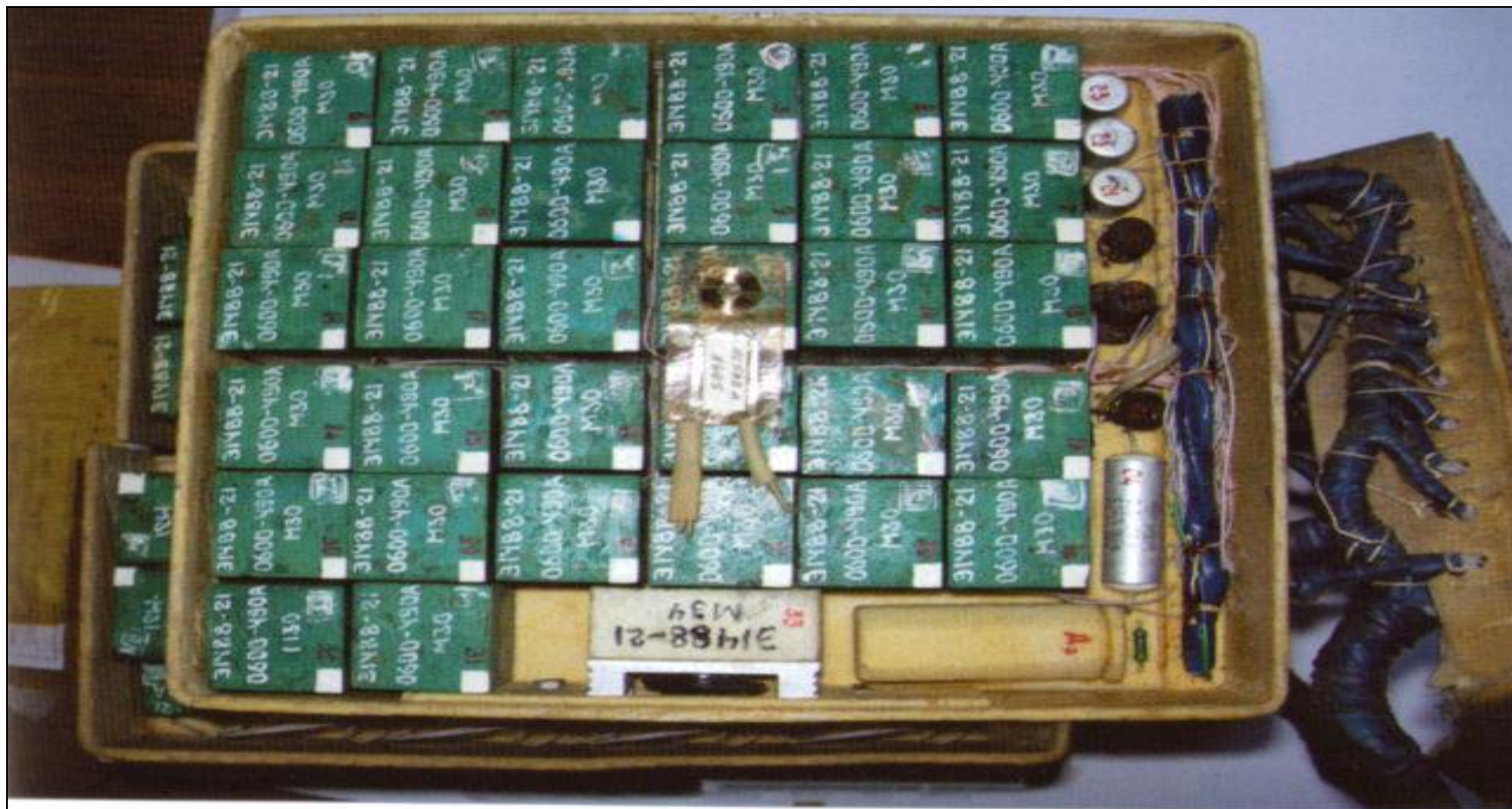
Платы технологического комплекта БЦВМ «Вычислитель»
