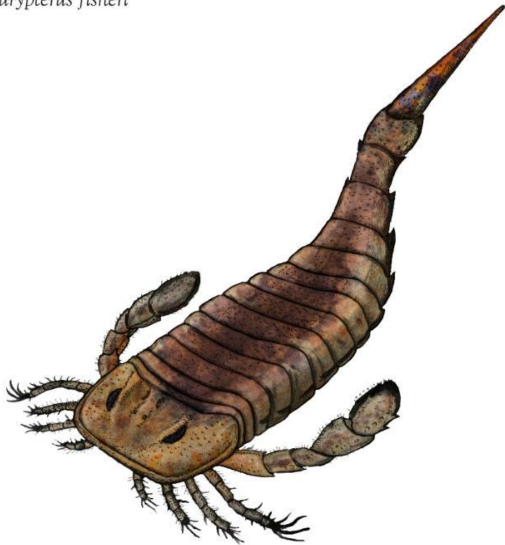
Eurypterus fisheri
