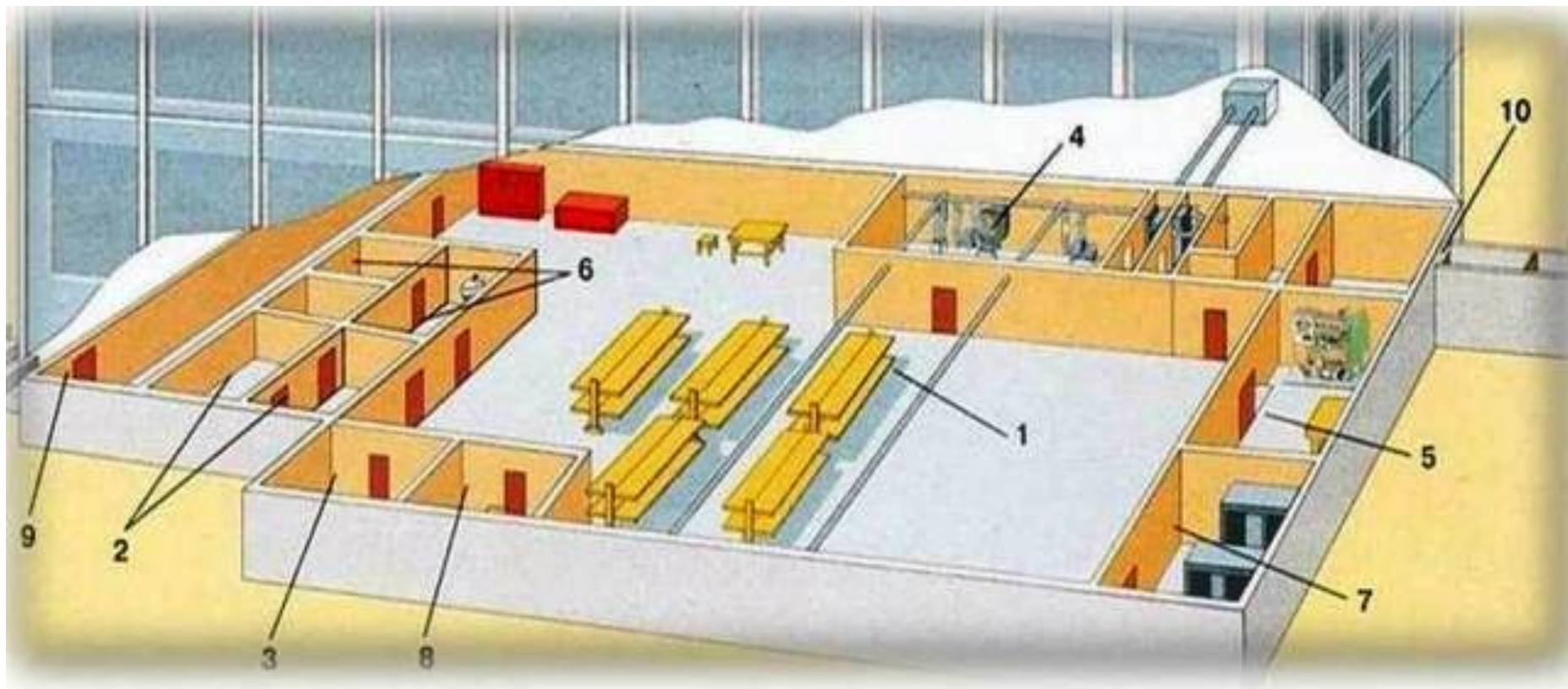
План убежища: 1—помещение для укрываемых; 2—пункт управления 3—медицинский пункт (может не устраиваться); 4—фильтровентиляционная камера 5—помещение дизельной электростанции; 6—санитарный узел; 7—помещение для GSM и электрощитовая; 8—помещение для продовольствия (может не устраиваться); 9—вход с тамбуром; 10—аварийный выход с тамбуром.
