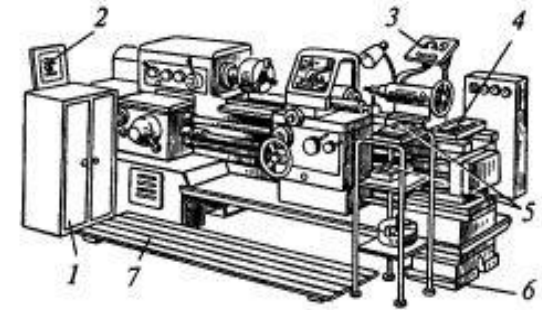
Рис. 4.5. Планировка рабочего места токаря:
