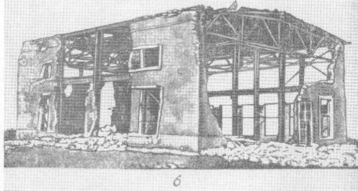
Рис. IV-19. Промышленное здание с металлическим каркасом, получившее сильное разрушение: a — до взрыва; б — после взрыва
