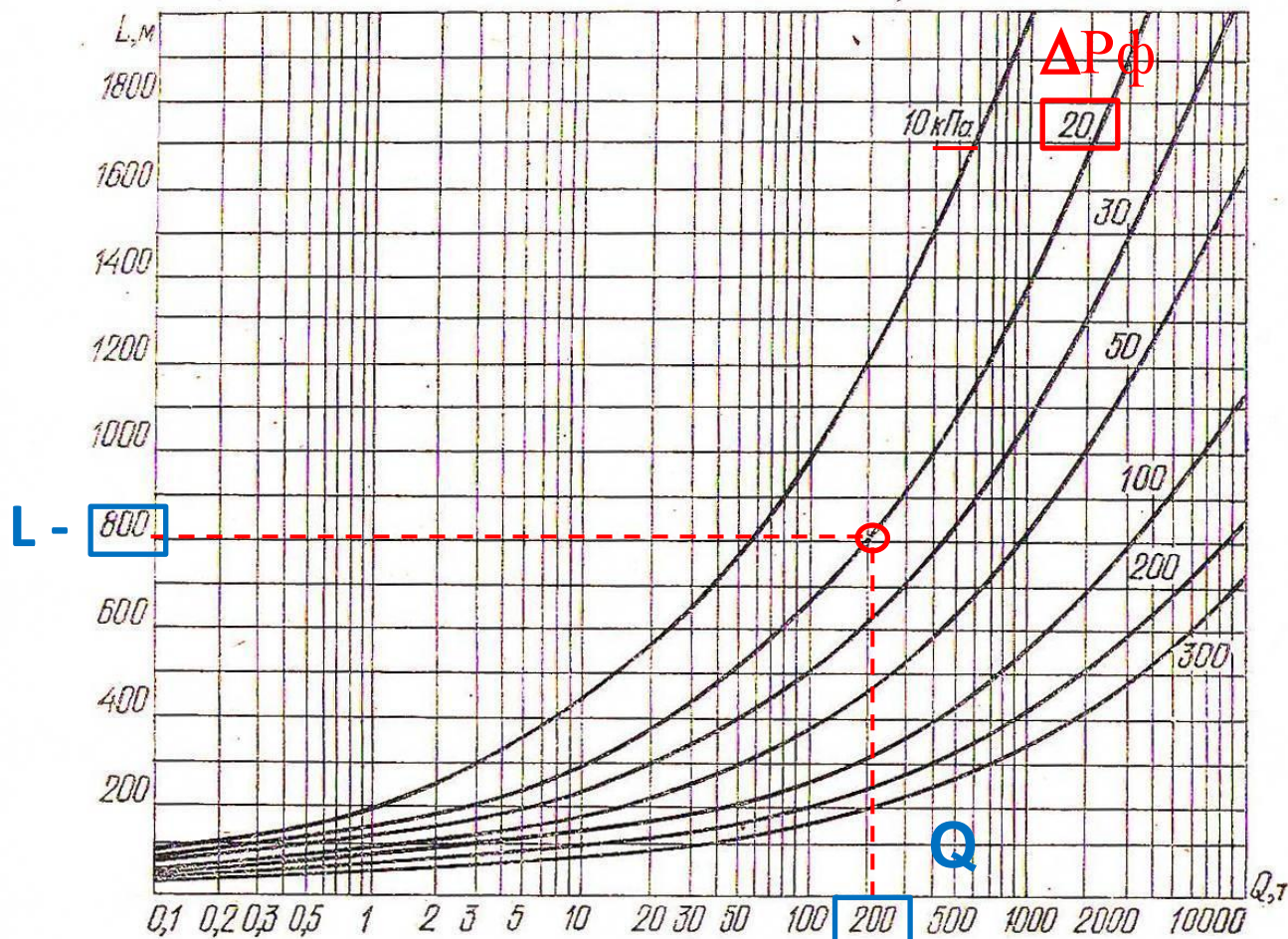
Рис. 10.2. Зависимость радиуса внешней границы зоны действия избыточного давления от количества взрывоопасной газовой смеси
