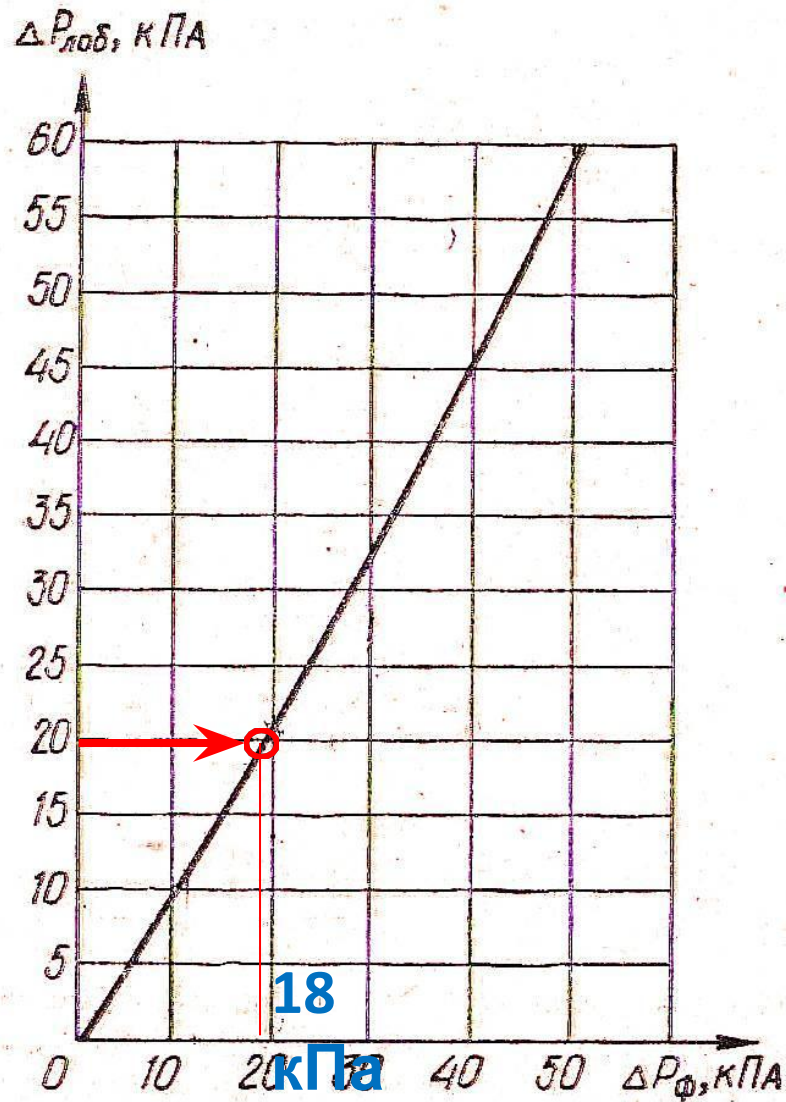
Рис. 8.6. Зависимость избыточного лобового давления \Delta P_{\text{л\o b}} от избыточного давления ударной волны \Delta P_{\phi}
