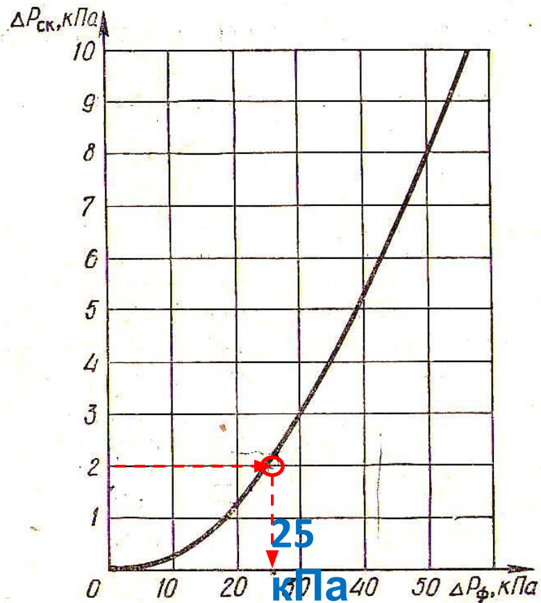
Рис. 8.3. Зависимость скоростного напора \Delta P_{ск} от избыточного давления ударной волны \Delta P_{\phi}
