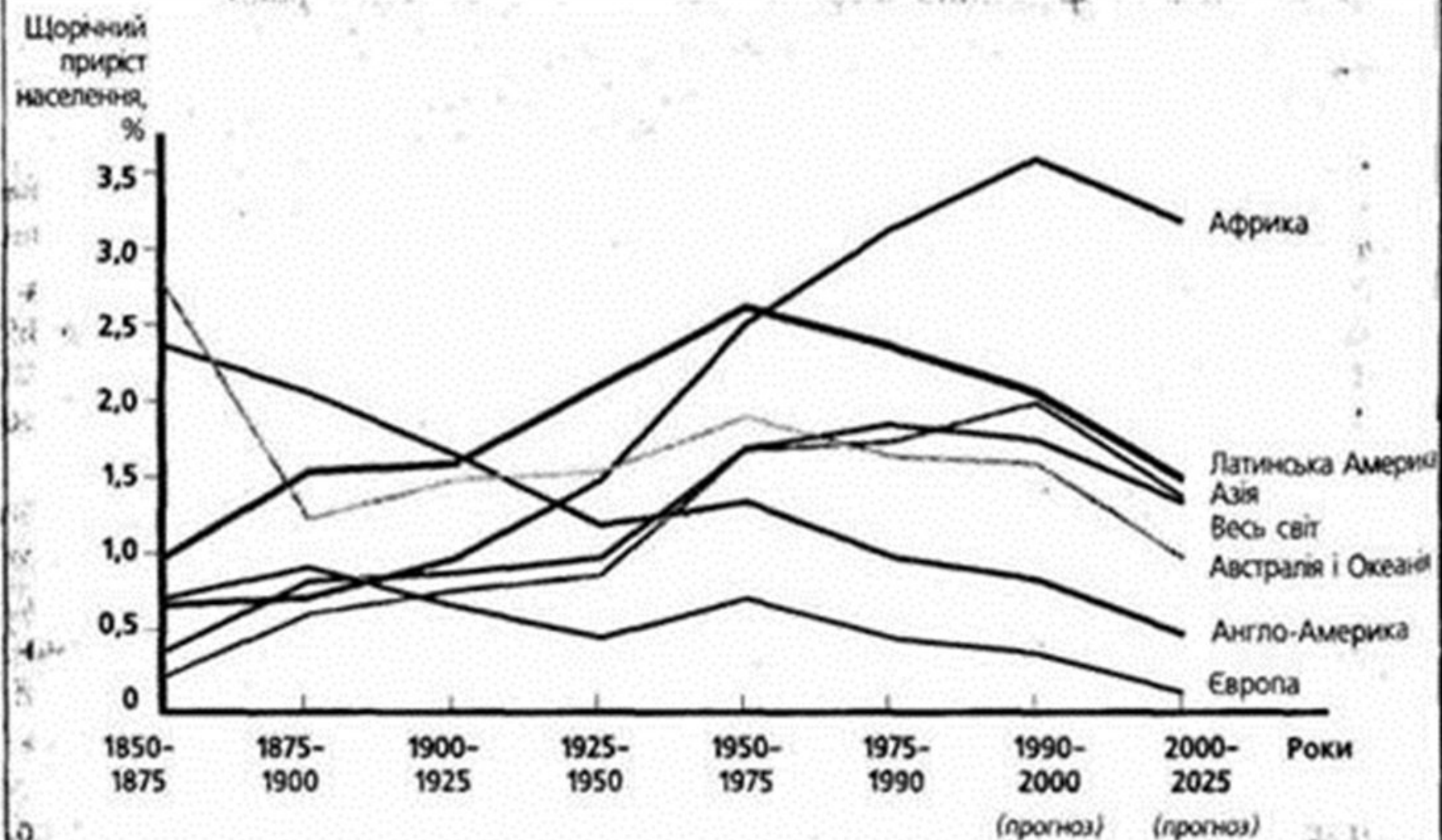
Мал. 41. Динаміка природного руху населення в історико-географічних регіонах світу
