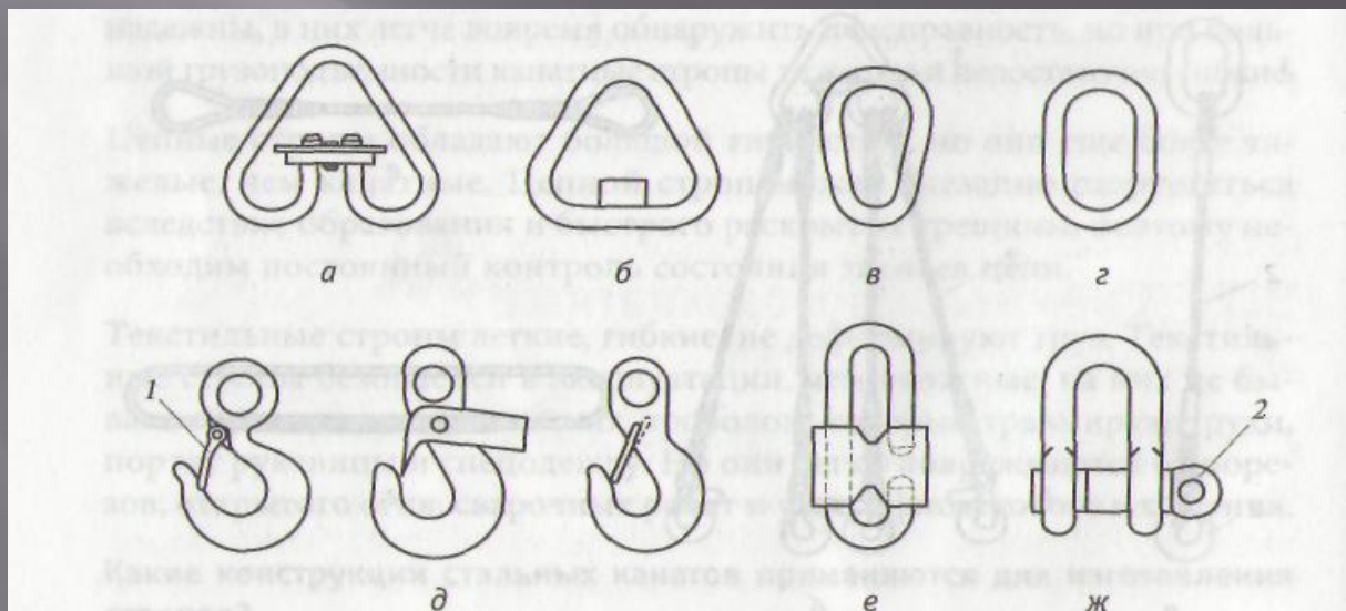
Рис. 3.8. Звенья стропов:
