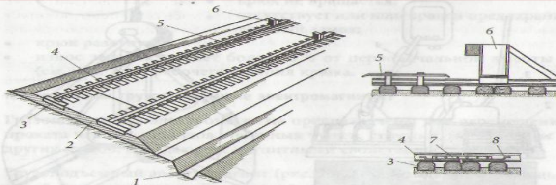
Рис. 2.14. Крановый путь:
