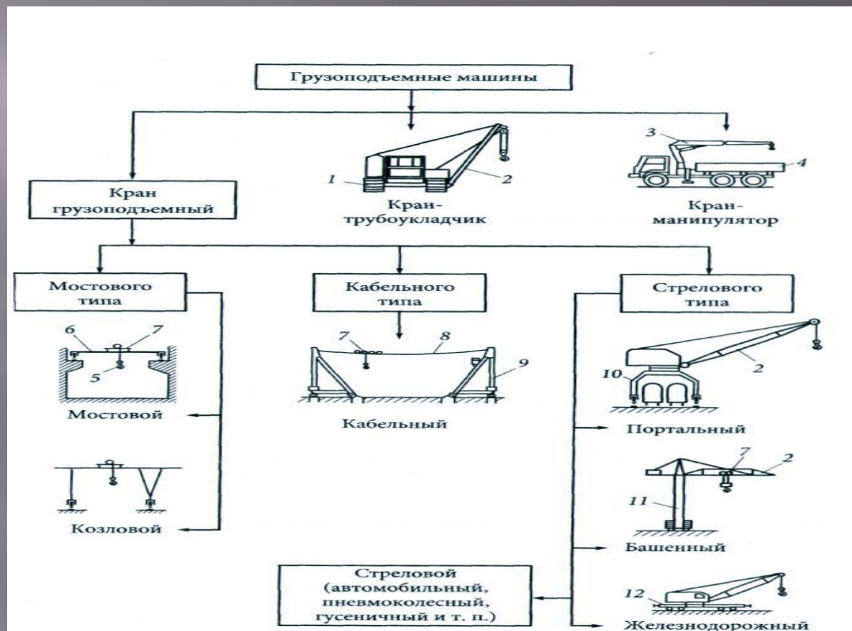
ис. 2.1. Грузоподъемные машины:
