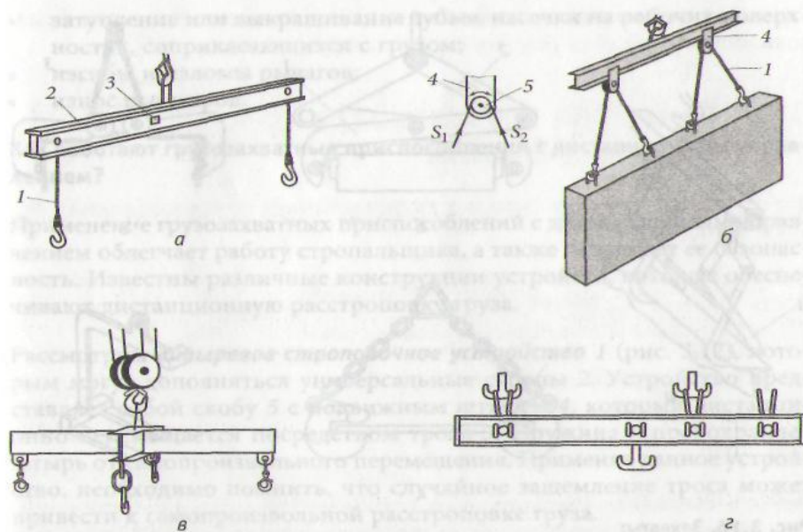
Рис. 3.15. Траверсы:
