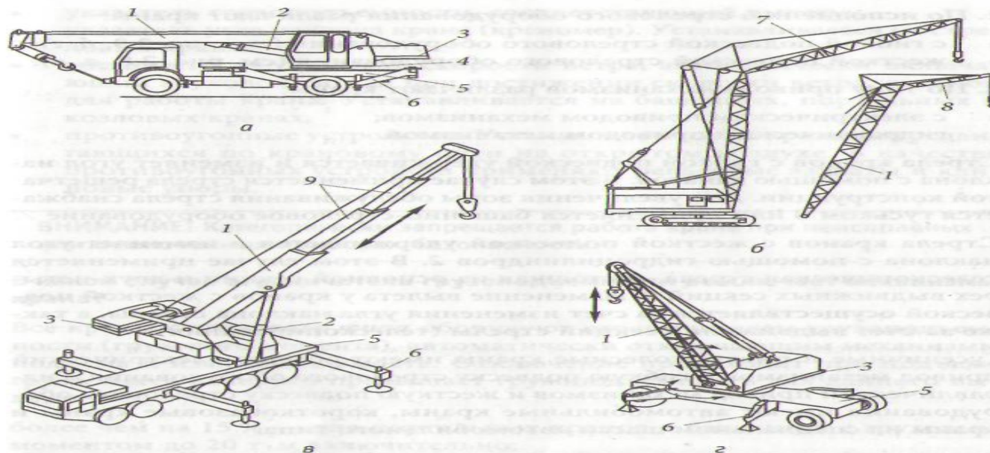
Рис. 2.8. Стреловые краны:
