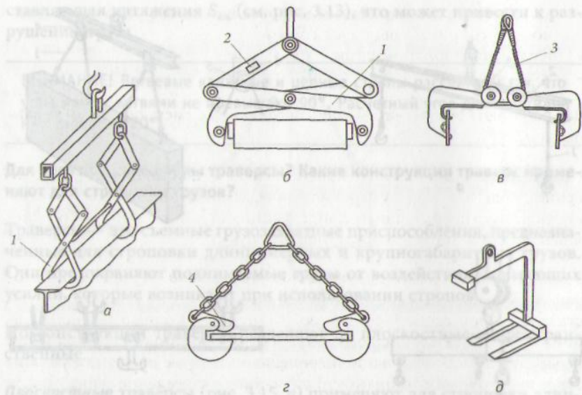
Рис. 3.16. Захваты:
