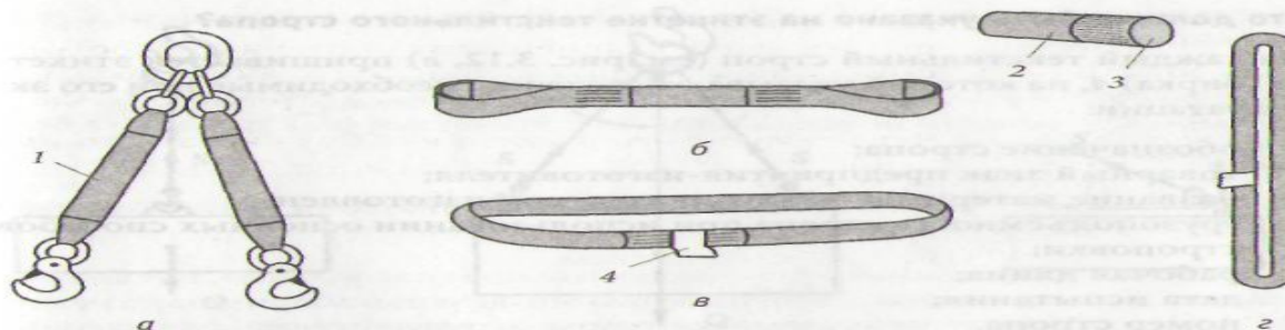
Рис. 3.12. Текстильные стропы:
