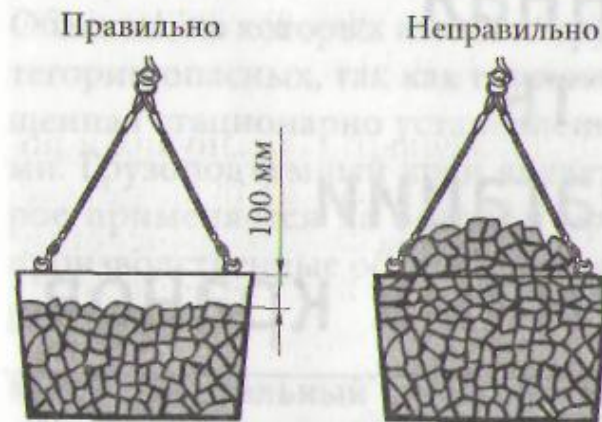
Рис. 3.23. Заполнение тары
