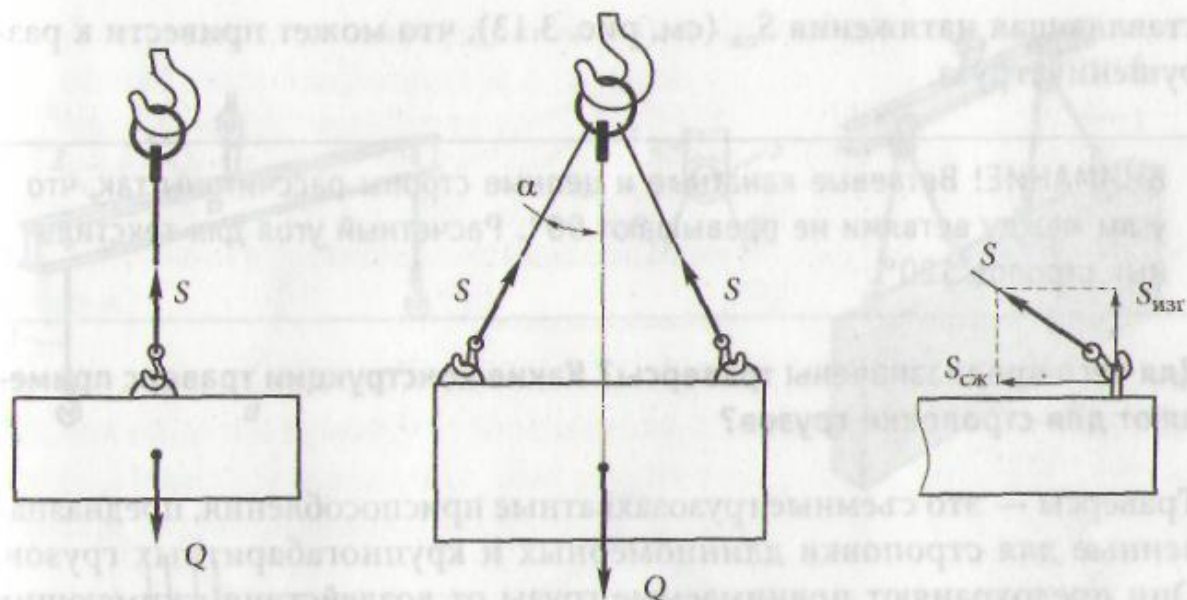
Рис. 3.13. Определение натяжения ветвей стропы:
