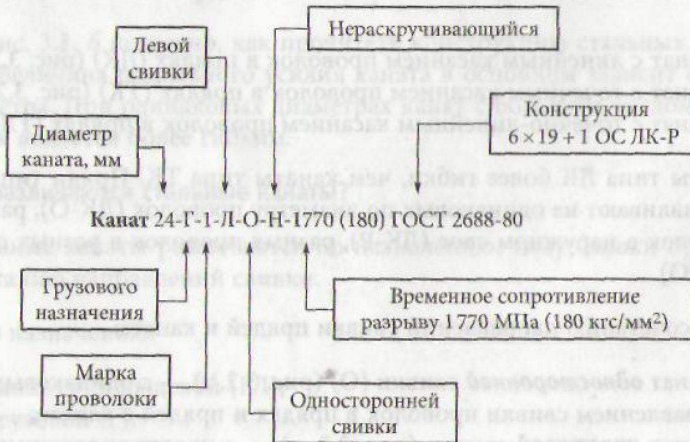
Рис. 3.3. Условное обозначение стального каната
