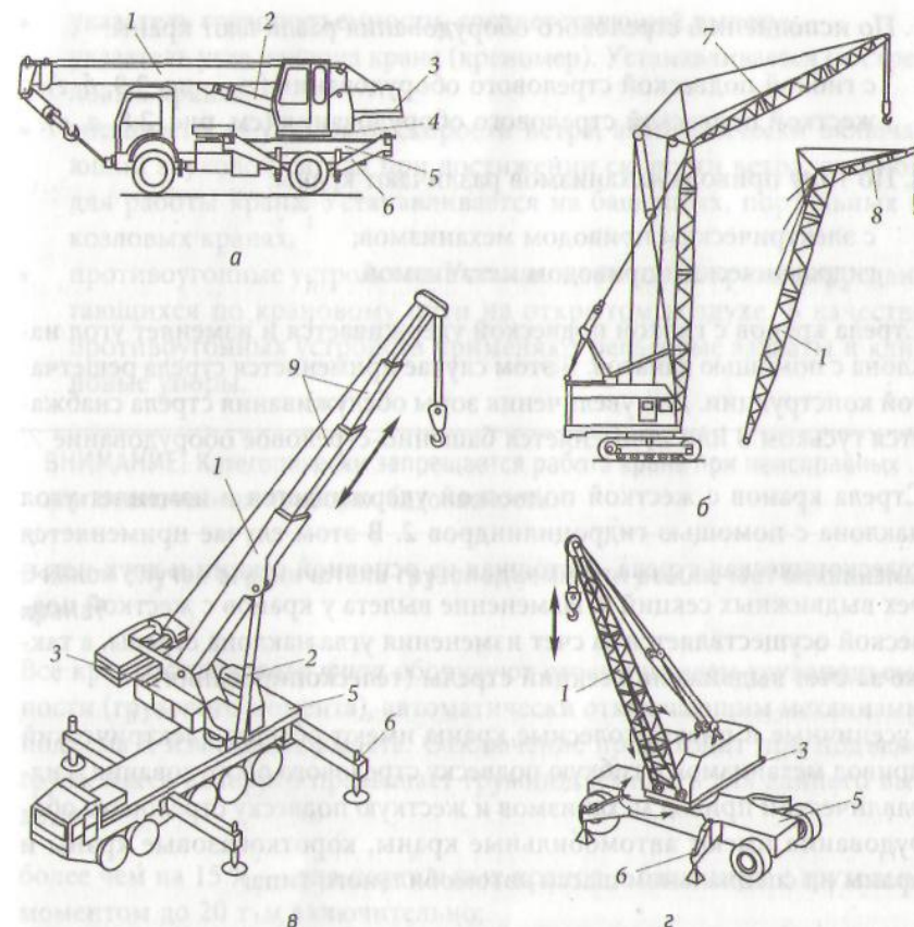
Рис. 2.8. Стреловые краны:
