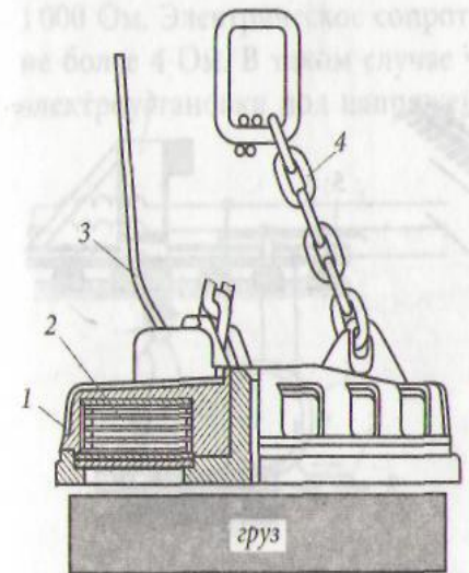
Рис. 2.12. Грузоподъемный электромагнит: 1 — корпус; 2 — катушка; 3 — кабель; 4 — цепь
