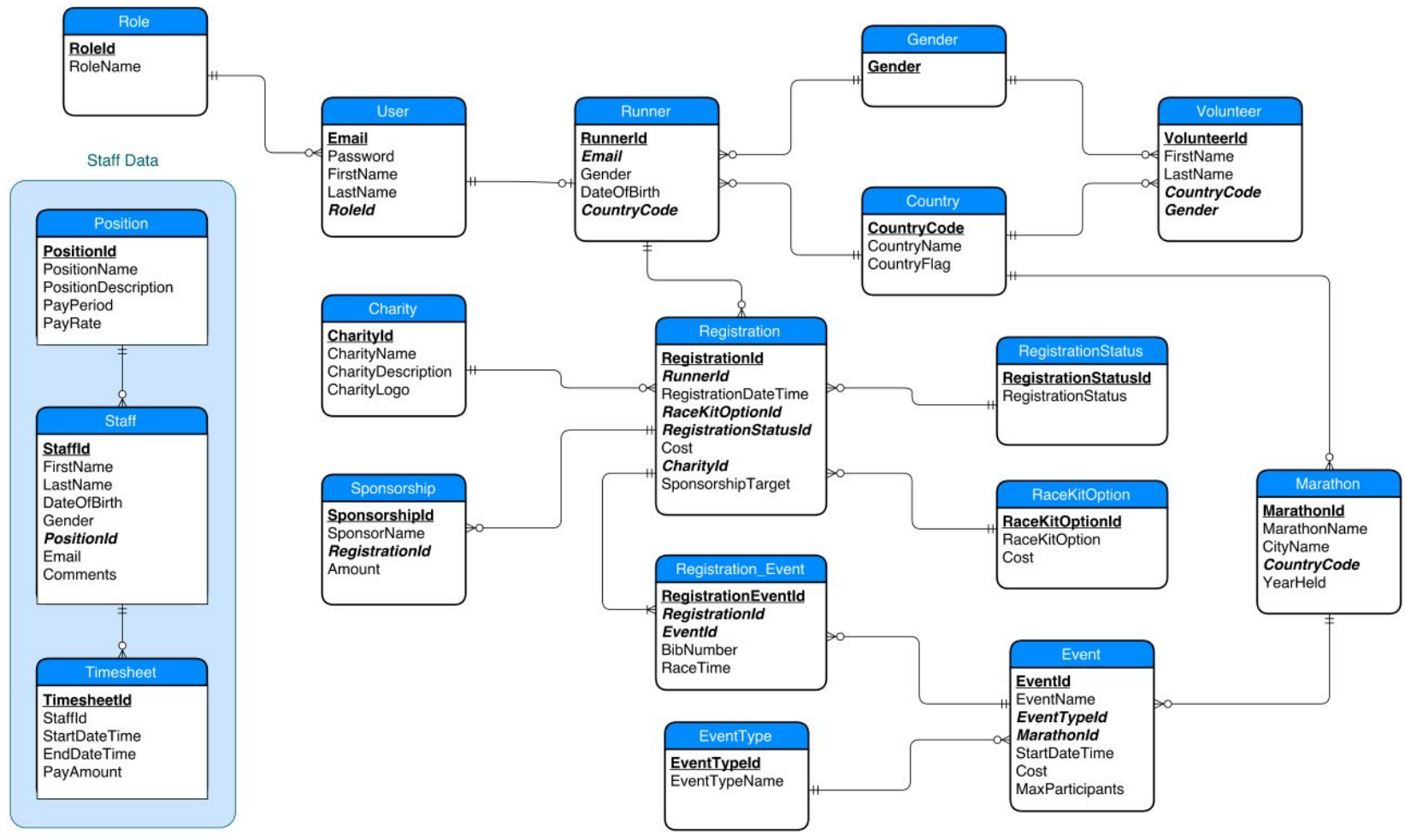
Диаграмма «Сущность-связь»
