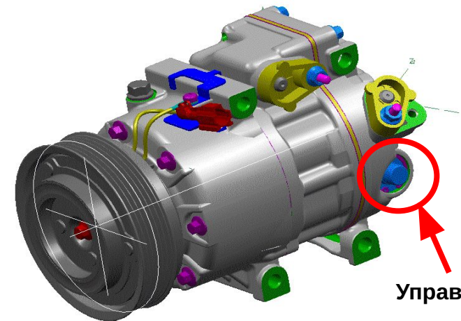
Компрессор переменного объёма (NF)
