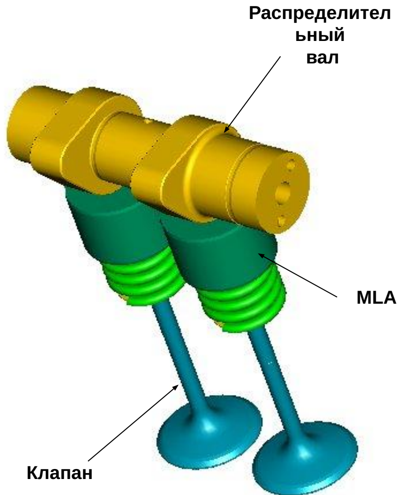
Θ/λ-двигатель
