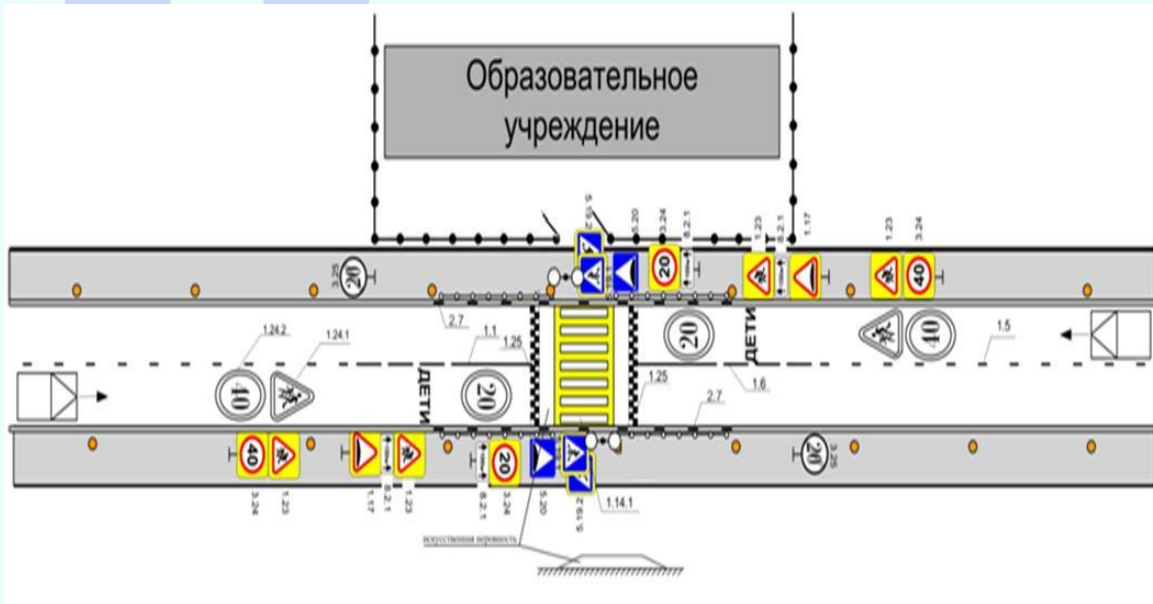
Схема размещения технических средств ОДД на подходах к образовательным учреждениям – ТИП 1
