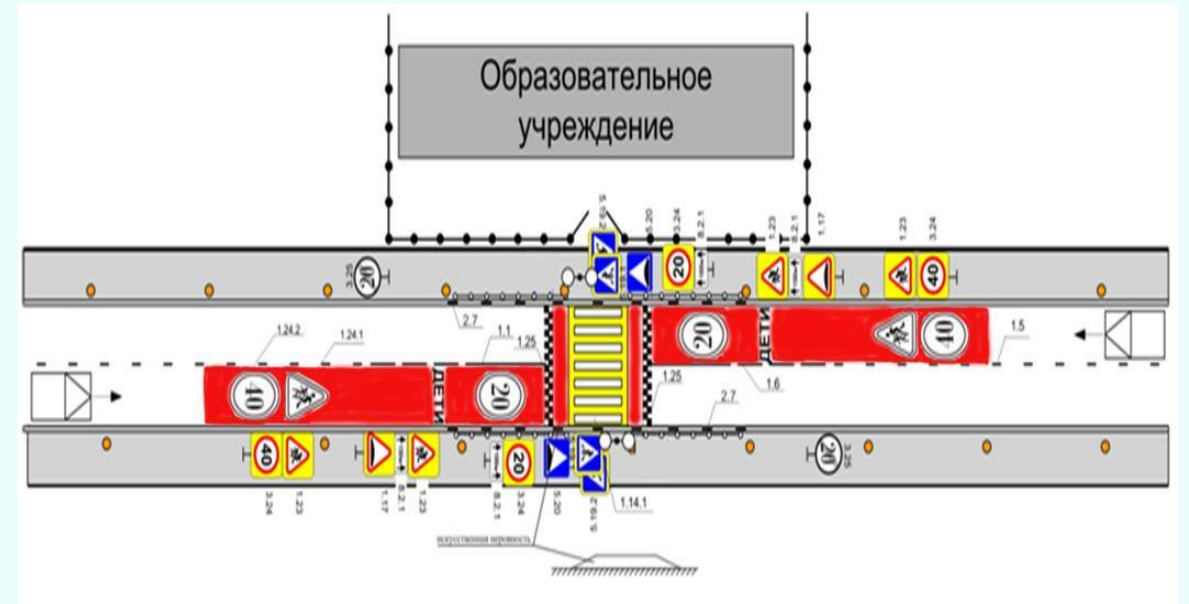
Усовершенствованная схема размещения технических средств ОДД на подходах к образовательным учреждениям – ТИП 1-доп (цветовое зонирование, лазерные стены, светодиодные катафорты)
