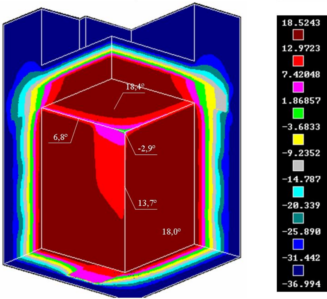
Общий вид распределения температур расчетного фрагмента узла сопряжения наружной стены с плитами чердачного перекрытия при отсутствии в монолитном ж/б поясе термовкладышей
