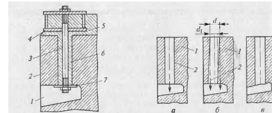
Рис. 9.3. Колодец в фундаменте для установки фундаментных болтов: 1 — ниша; 2 — фундамент; 3 — фундаментный болт; 4 — фундаментная плита; 5 — цементная подливка; 6 — колодец; 7 — анкерная плитка
