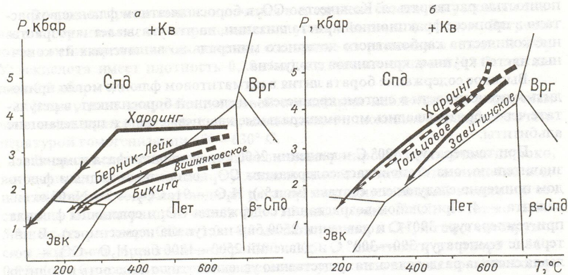
Рис. 7.1. Пути процесса кристаллизации на P - T -диаграмме, определяемые ассоциацией литневых алюмосиликатов и кварца [London, 1984].
