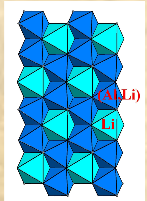
Лепидолит-2M 1
