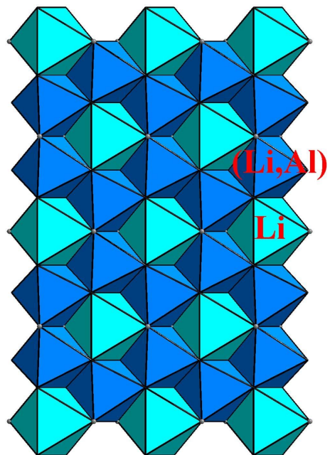
Полилитионит
