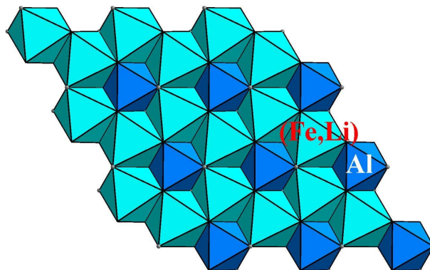
Циннвальдит
