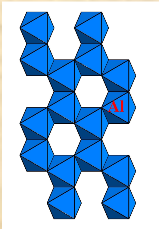
Мусковит
