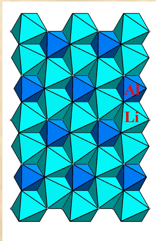
Лепидолит-1M
