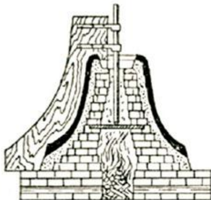
Стадии изготовления формы колокола согласно традиционной русской технологии.
