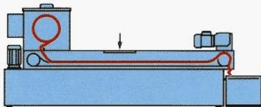
Гравитационный ленточный фильтр
