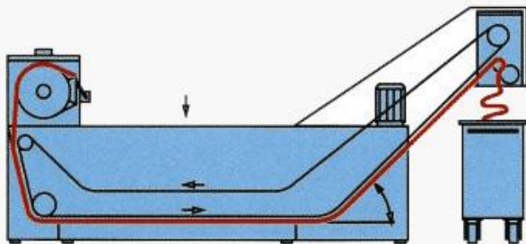
Вакуум-фильтр
