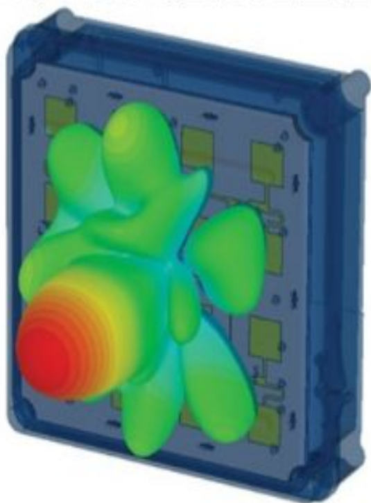
Vzorec Záření 4 x 4 Fázového Pole
