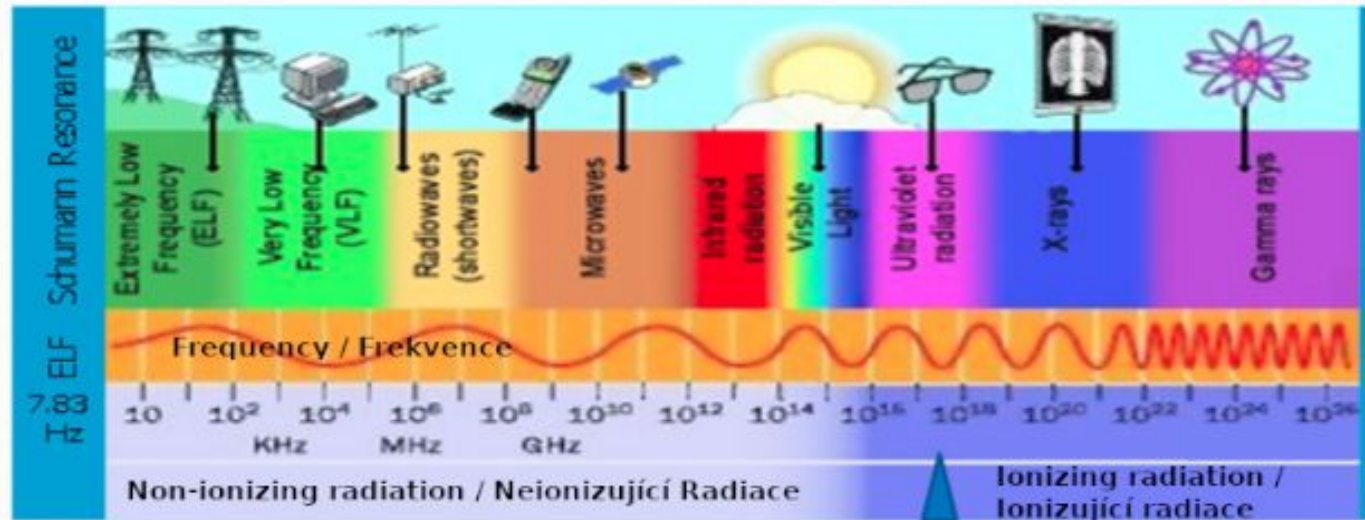
Electromagnetic spectrum - Elektromagnetické Spektrum
