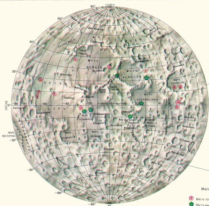
ВИДИМОЕ ПОЛУШАРИЕ ЛУНЫ
