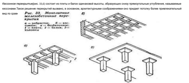
Рис. 33. Монолитные железобетонные перекрытия а - ребристые; б - кессонное; в - бесбалочное; 1 - плита; 2 - балка; 3 - колонна
