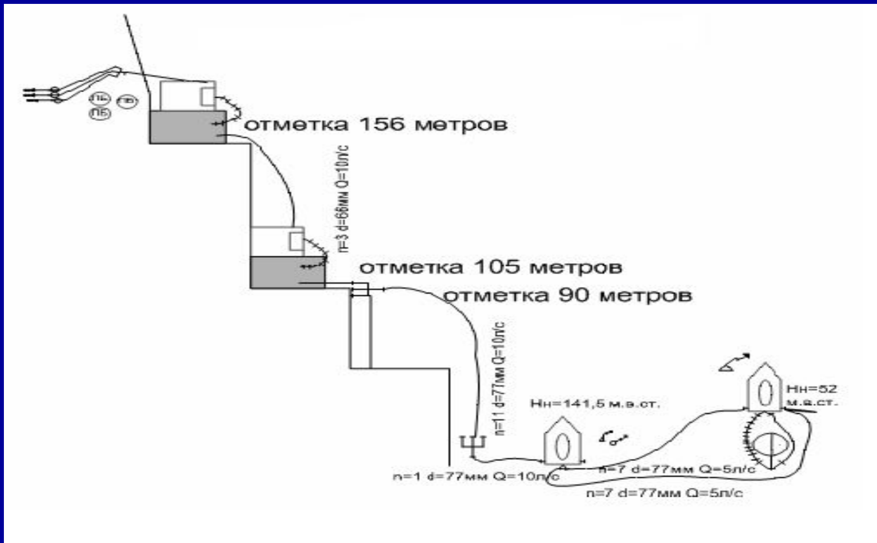
Рис. 2. Схема подачи огнетушащих средств на тушение пожара способом перекачки «из насоса через промежуточную емкость» с помощью переносных мотопомп.
