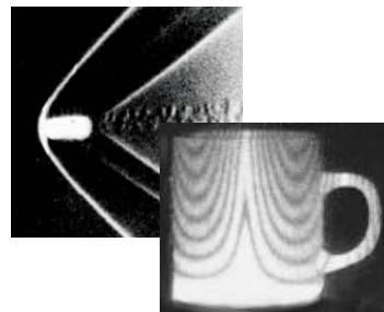
Картинки мех. напряжений и плотностей
