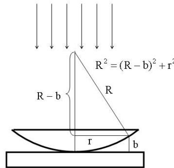
Исаак Ньютон Корпускулярная теория света не позволила объяснить возникновение колец
