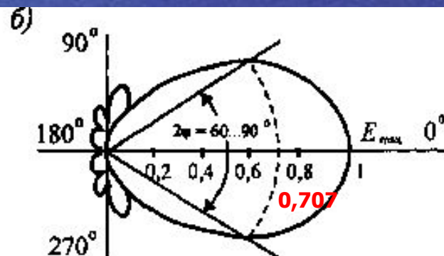
полуромбическая антенна
