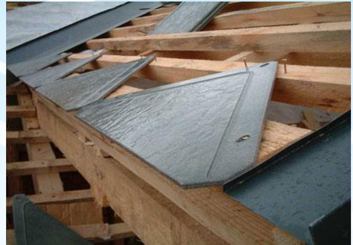
Монтаж первого ряда плиток формата 40x40.
